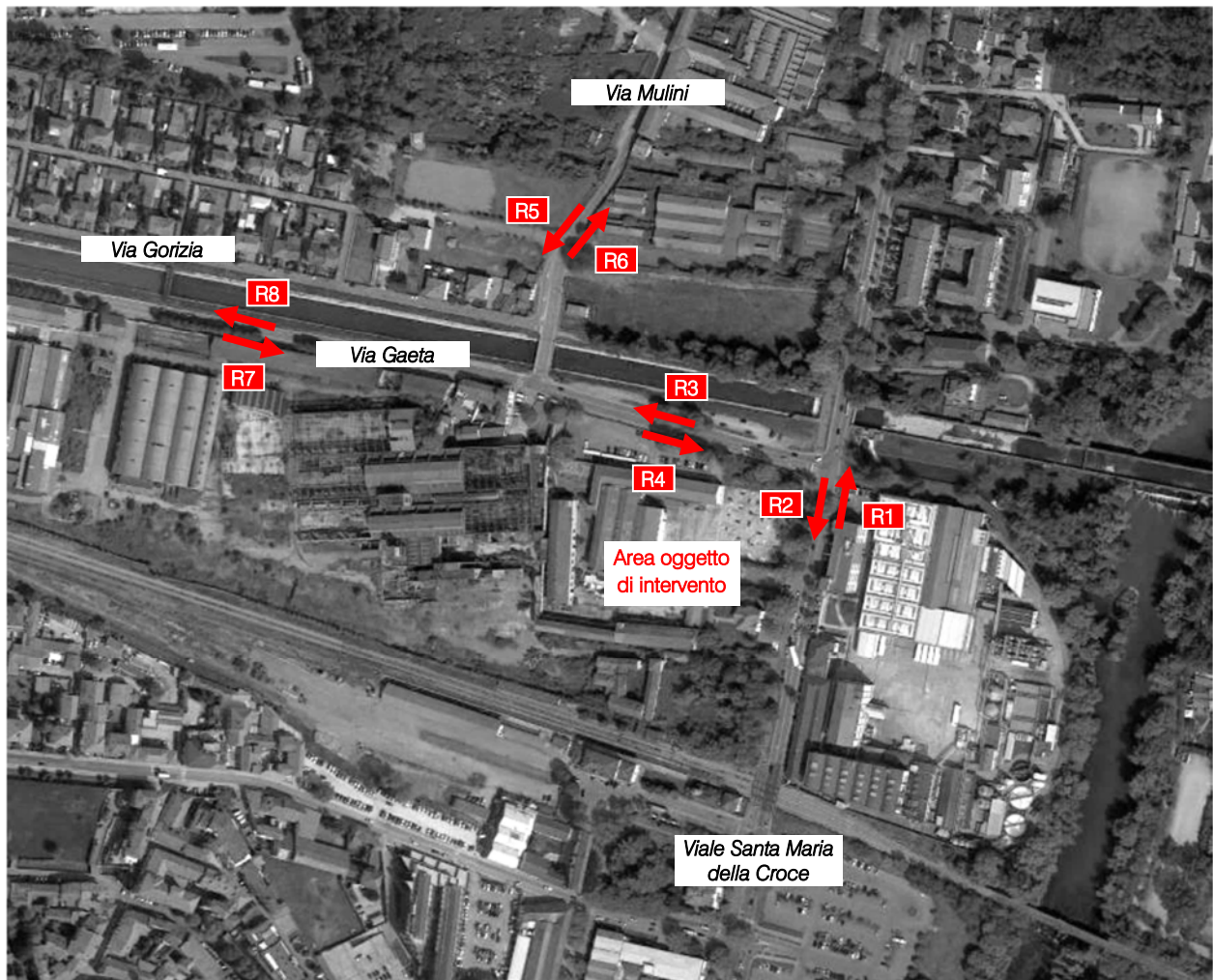
Figura B.1 – Posizionamento apparecchiature radar
