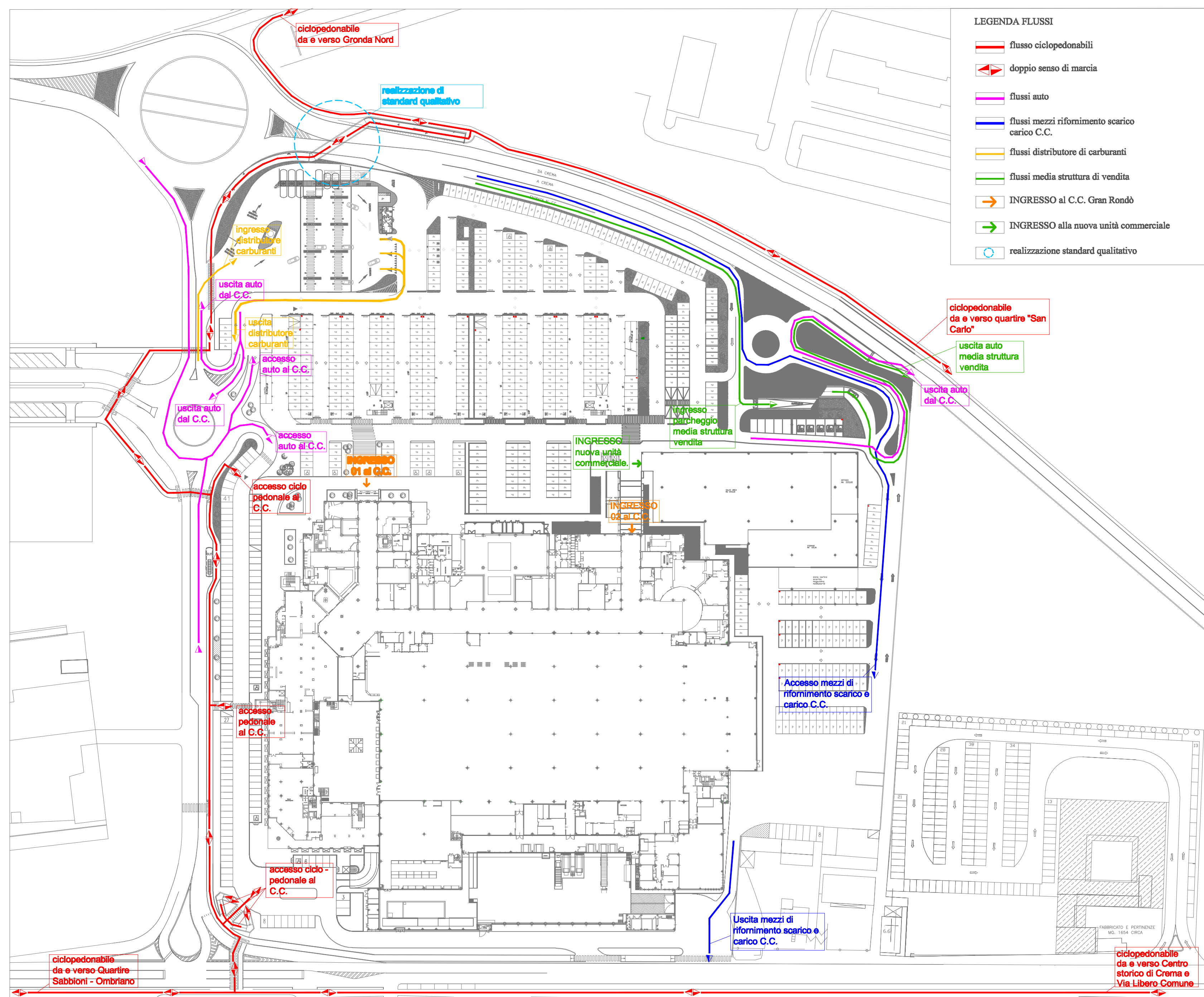
PLANIMETRIA STATO FUTURO FLUSSI VEICOLARI
