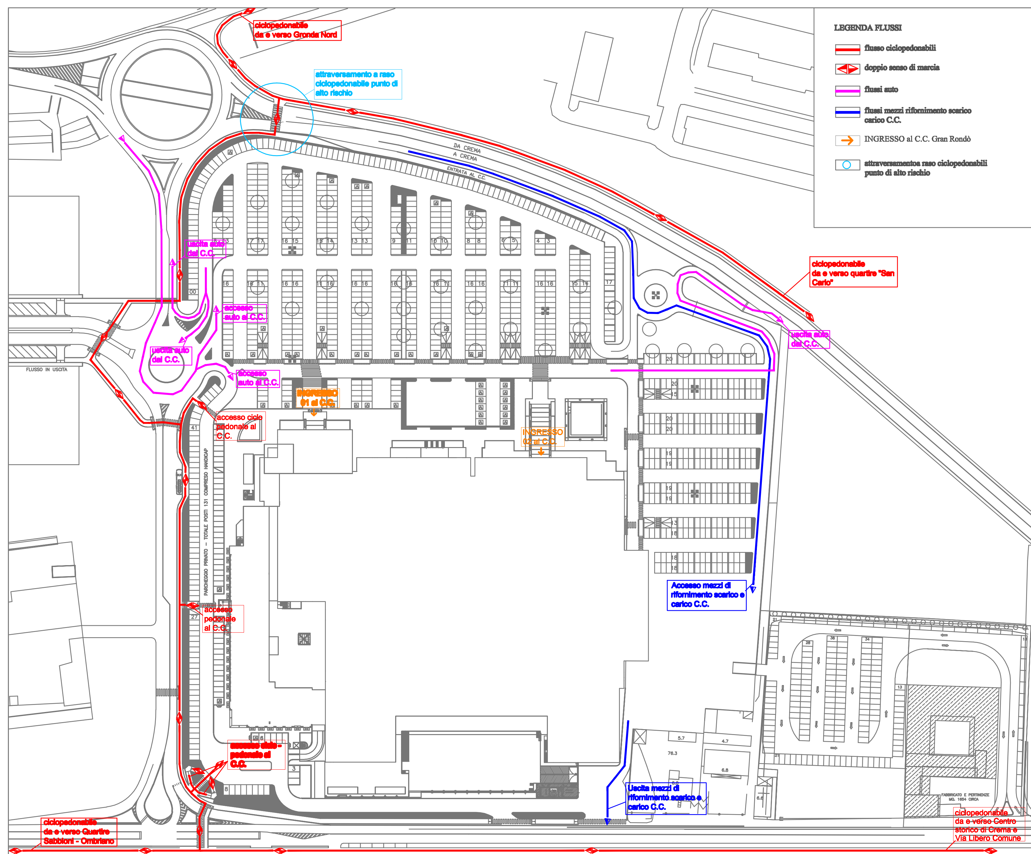
PLANIMETRIA STATO DI FATTO FLUSSI VEICOLARI
