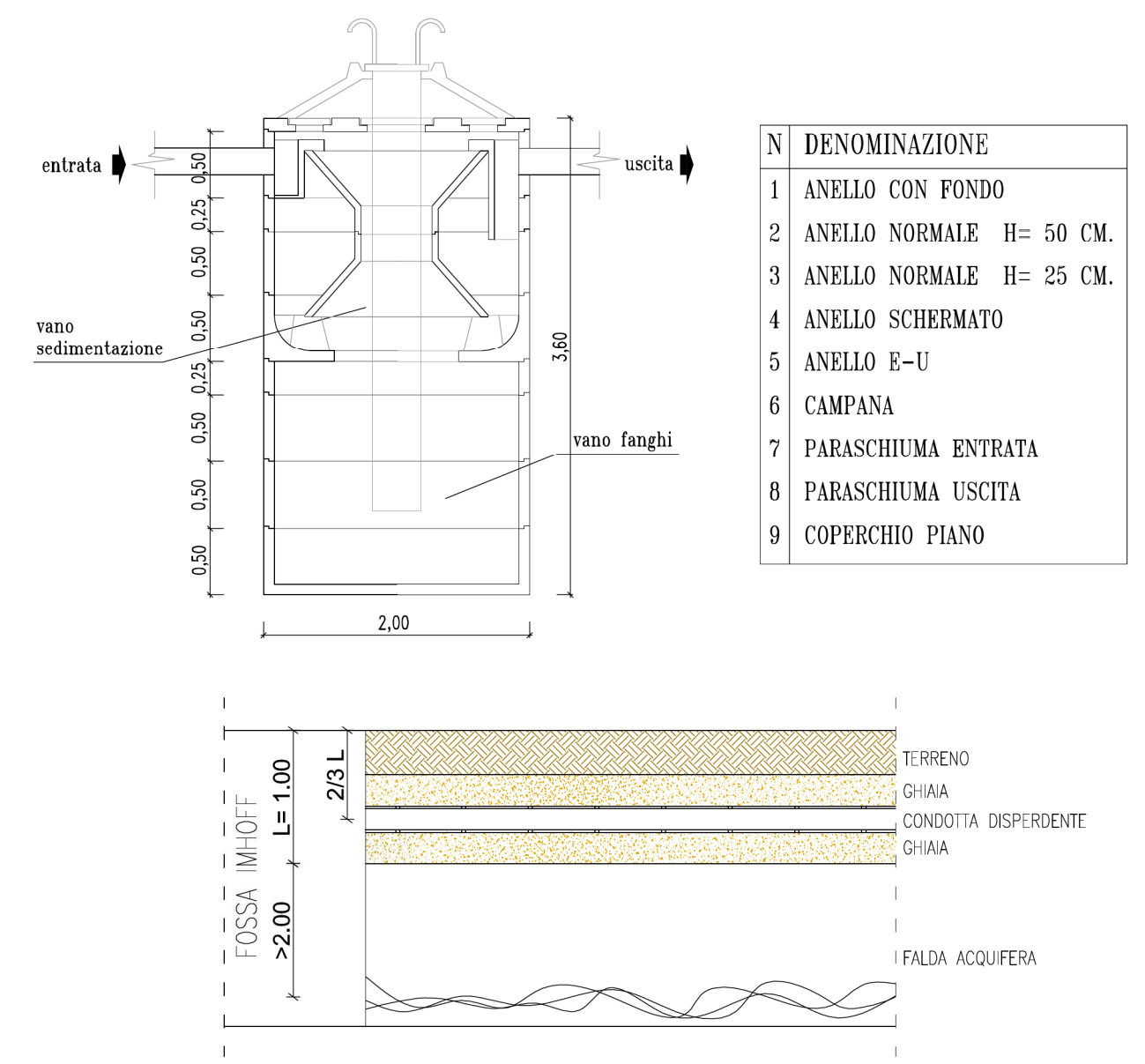
FOSSA BIOLOGICA (IMHOFF) PARTICOLARE FOSSA BIOLOGICA E CONDOTTA DISPERDENTE - SCALA 1:50
